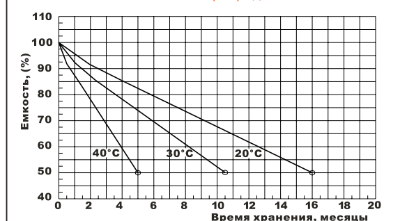
Саморазряд
