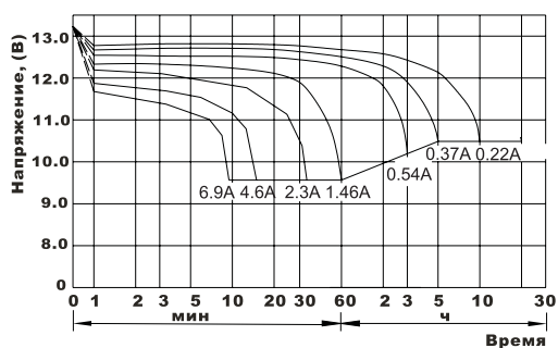
Разрядные характеристики (25°C)
