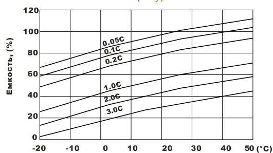
Влияние температуры на емкость
