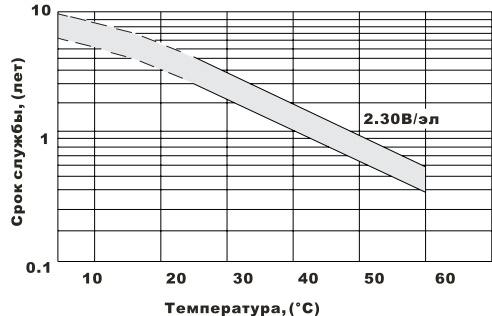
Влияние температуры на срок службы
