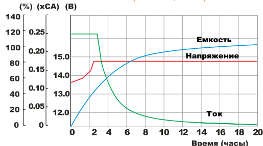
Заряд постоянным напряжением (0.25СА, 25°C)
