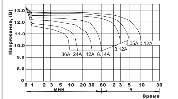
Разрядные характеристики (25°C)
