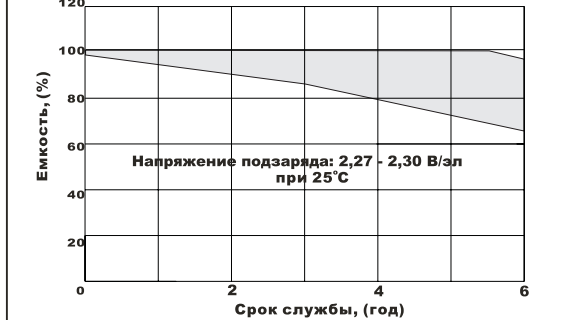
Срок службы в буферном режиме
