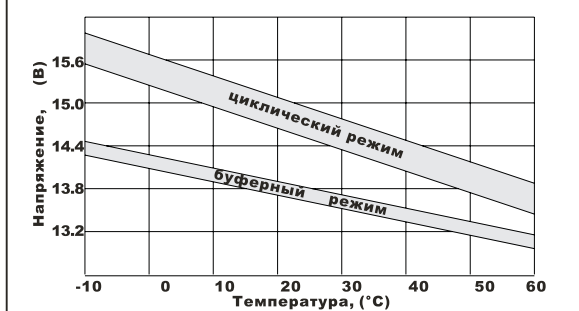
Влияние температуры на напряжение заряда
