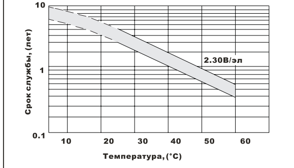
Влияние температуры на срок службы
