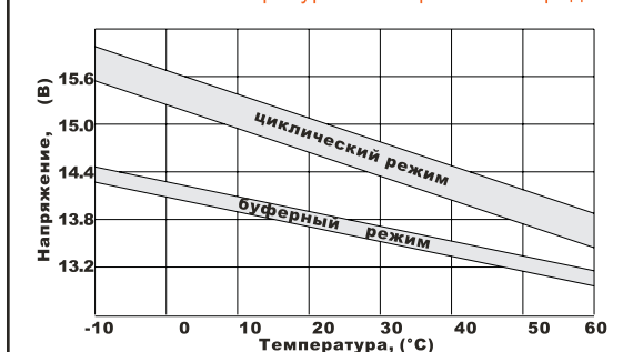
Влияние температуры на напряжение заряда
