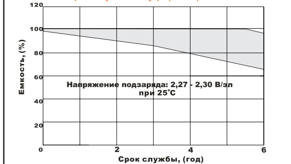
Срок службы в буферном режиме
