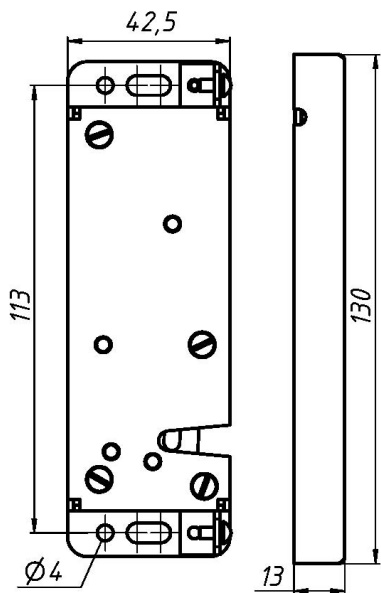
Рис.5 Корпус замка
