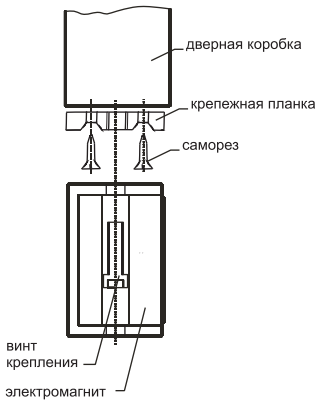
Рис. 2. Схема установки электромагнита M1-150, M1-200
