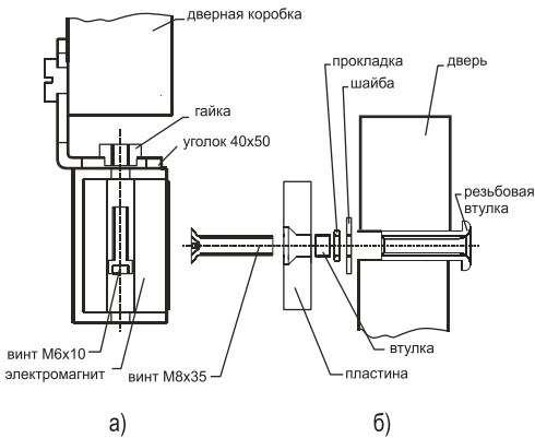
Рис. 1. Схема установки замка
