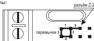
Рис.1 Положения переключки.
