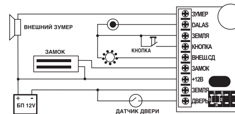
Рис.2 Схема подключения.
