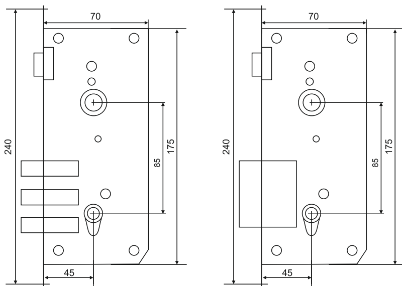
4. Установочные размеры ВЕКТОР-ЭМЗ
