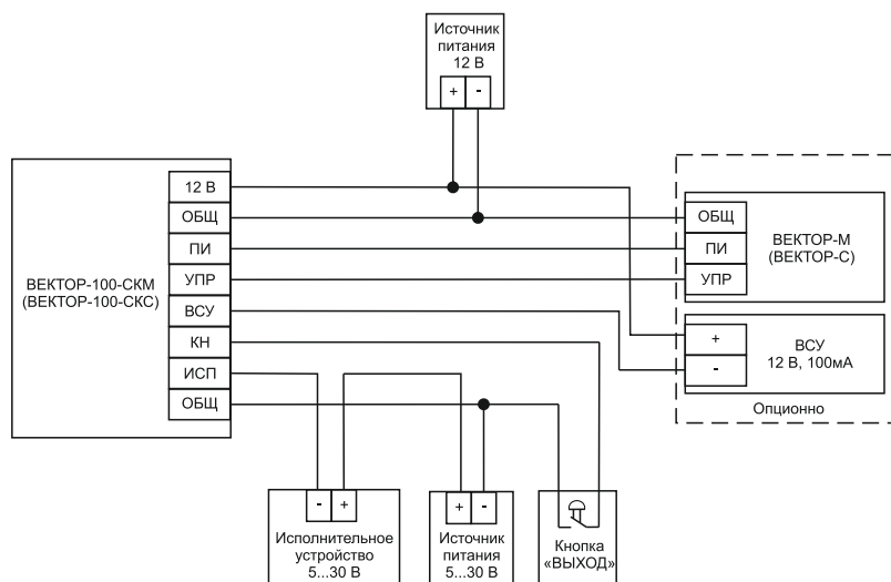
2. Схема соединений ВЕКТОР-100-СКМ (ВЕКТОР-100-СКС) при использовании исполнительного устройства с напряжением питания от 5 до 30 В.
