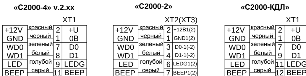
Рисунок 1. Схемы подключения к ПКП и контроллерам СКД (считыватель всегда слева)
