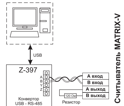
Рис.5 Схема подключения по RS-485.
