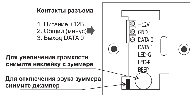
Рис.1 Схема подключения.
