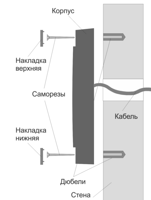
Рисунок 4. Крепление считывателя PNR-P19
