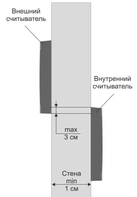
Рисунок 4. Крепление считывателей с разнесением по вертикали
