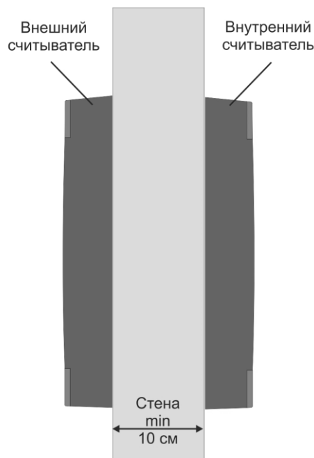
Рисунок 3. Крепление считывателей на одном уровне
