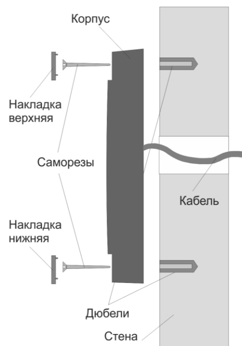
Рисунок 2. Крепление считывателя
