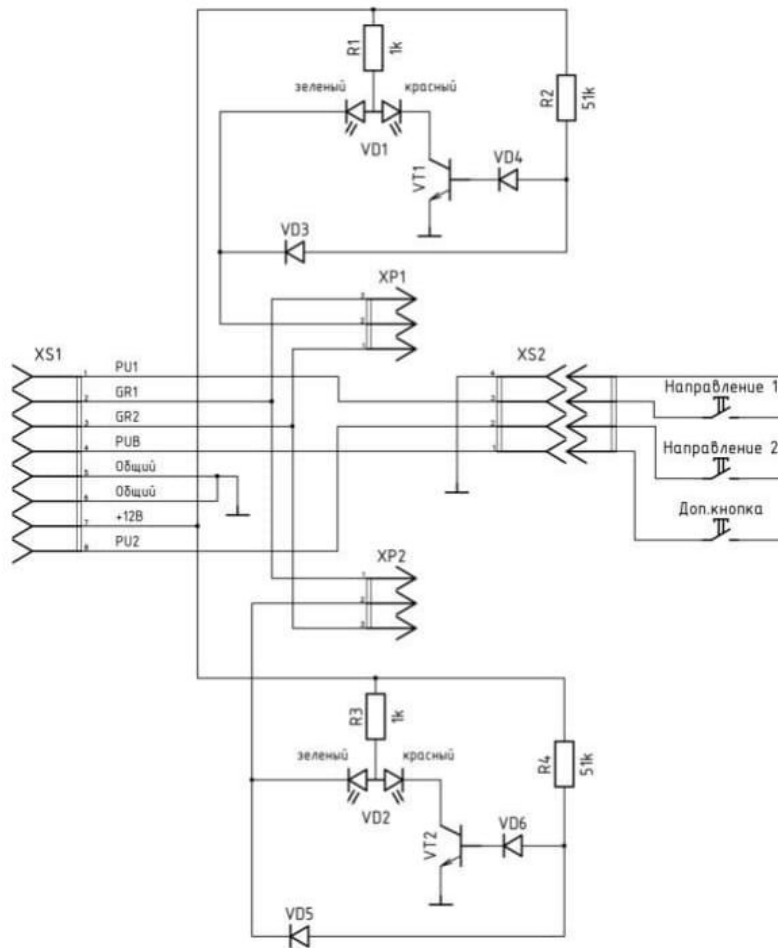
Схема электрическая принципиальная пульта дистанционного П2П-0-0Г
