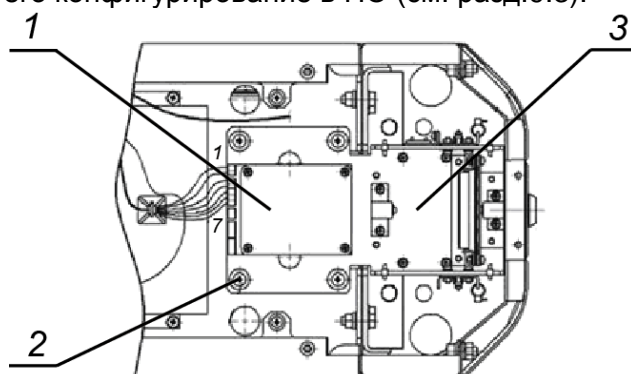
Рисунок 15. Механизм картоприемника
