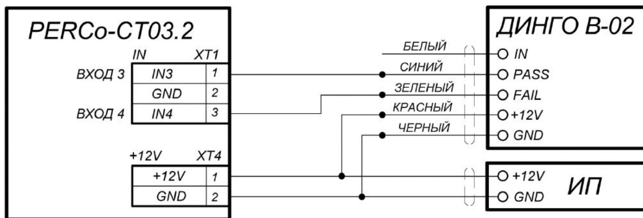
Рисунок 18. Схема подключения алкотестера «Динго В-02» (ООО СИМС-2)
