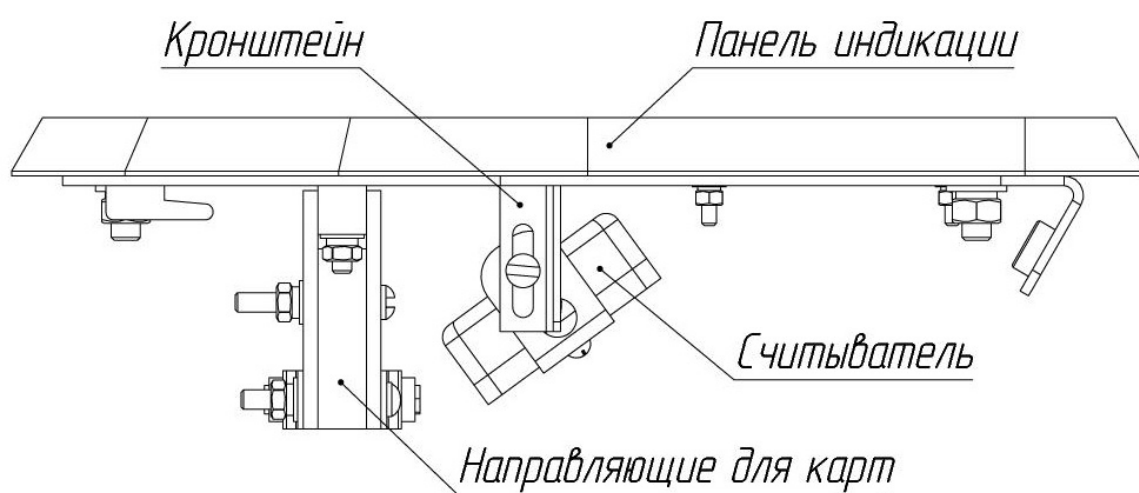
Рис. 17. Рекомендуемый вариант установки считывателя бесконтактных карт
