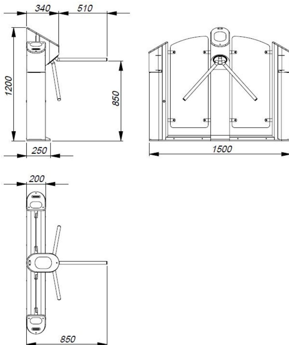
Рис. 2. Габаритные размеры турникета
