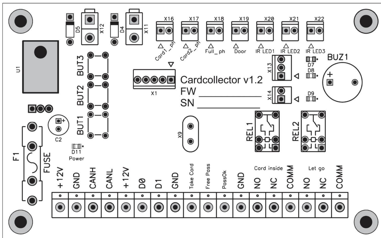
Рис. 14. Внешний вид платы картоприемника
