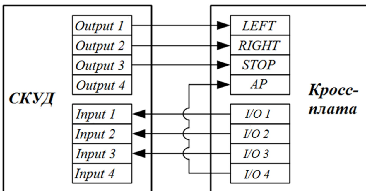
Рис. 12. Схема подключения ПУ к контроллеру СКУД
