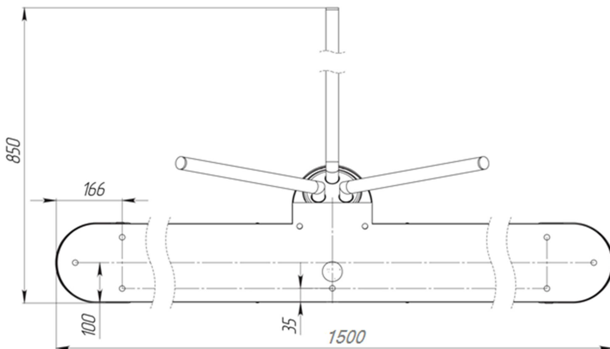
Рис. 21. Расположение монтажных отверстий относительно внешних габаритов турникета
