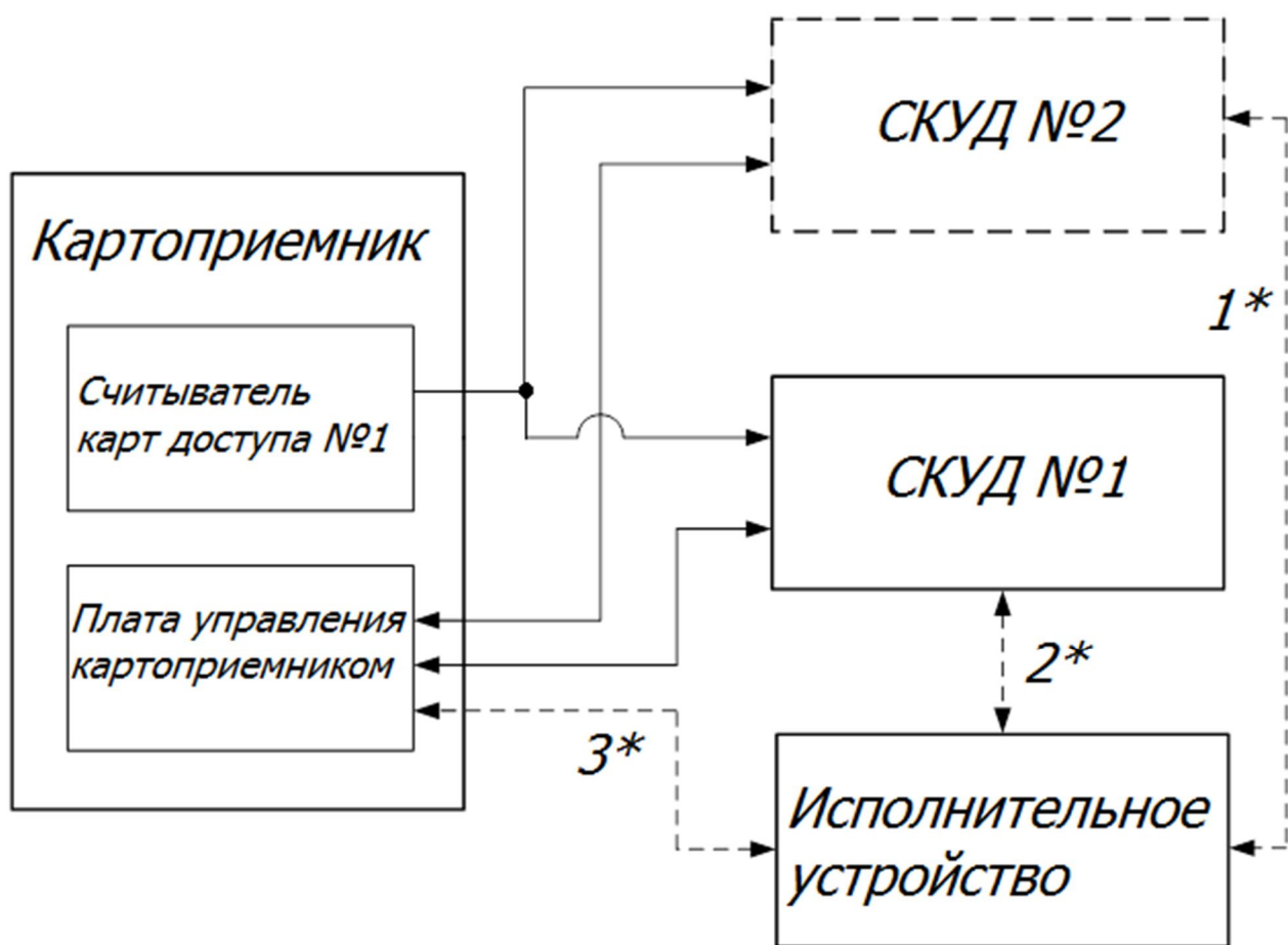
Рис. 19. Структурная схема №2
