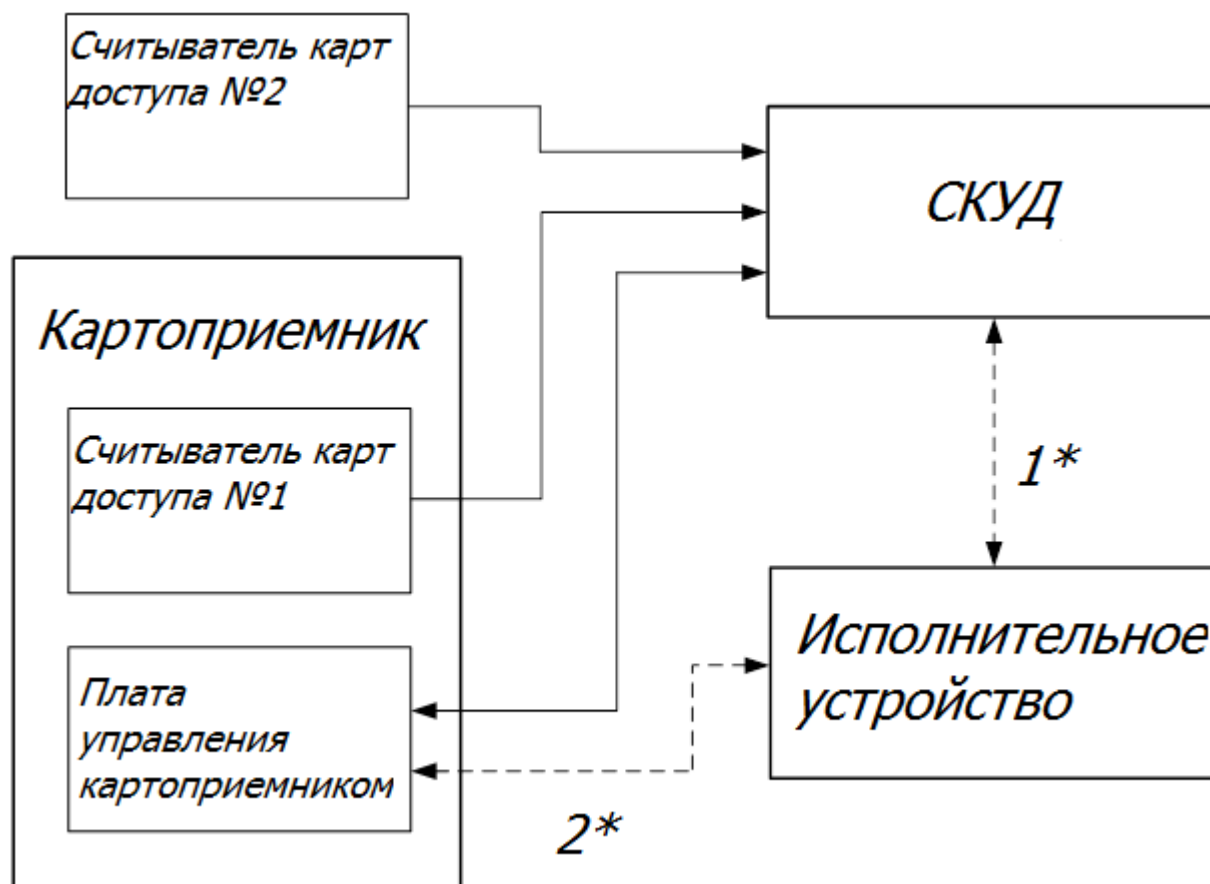
Рис. 18. Структурная схема №1
