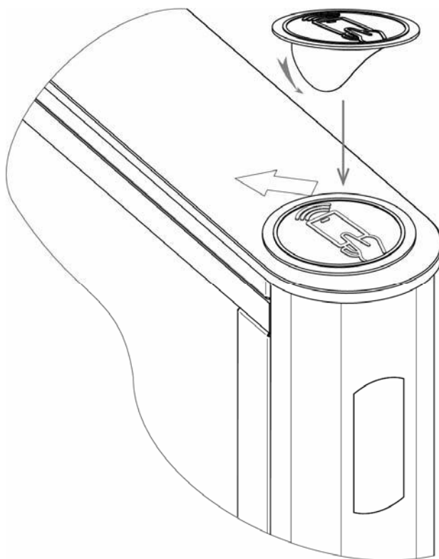
Рисунок 25. Наклеивание резиновой накладки на стеклянную крышку
