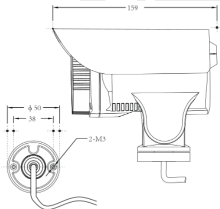
Рисунок 3 Размеры
