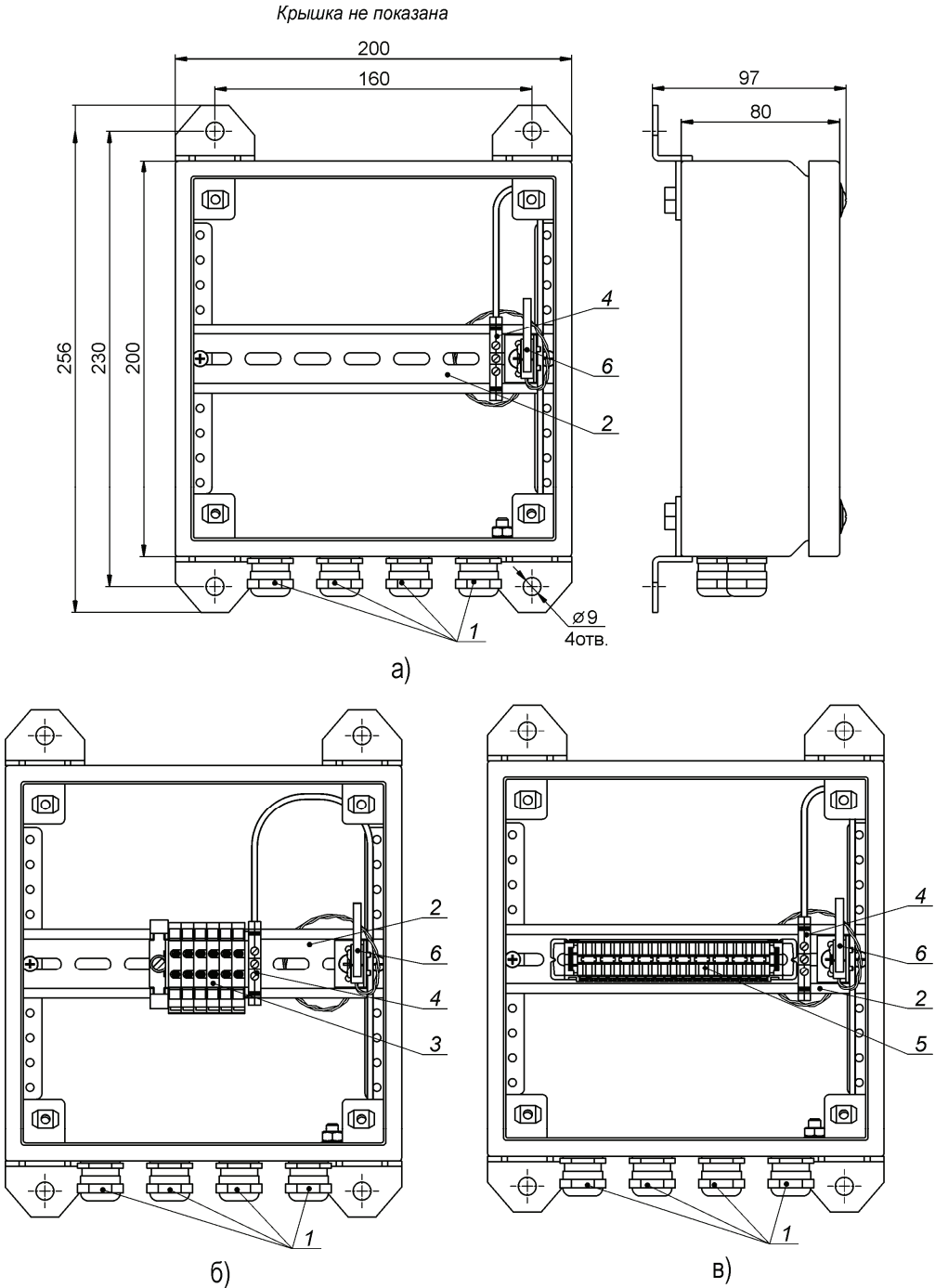
Рис.1 Устройство и габаритные размеры КМ-4 (а), КМ-5 (б) и КМ-6 (в)
