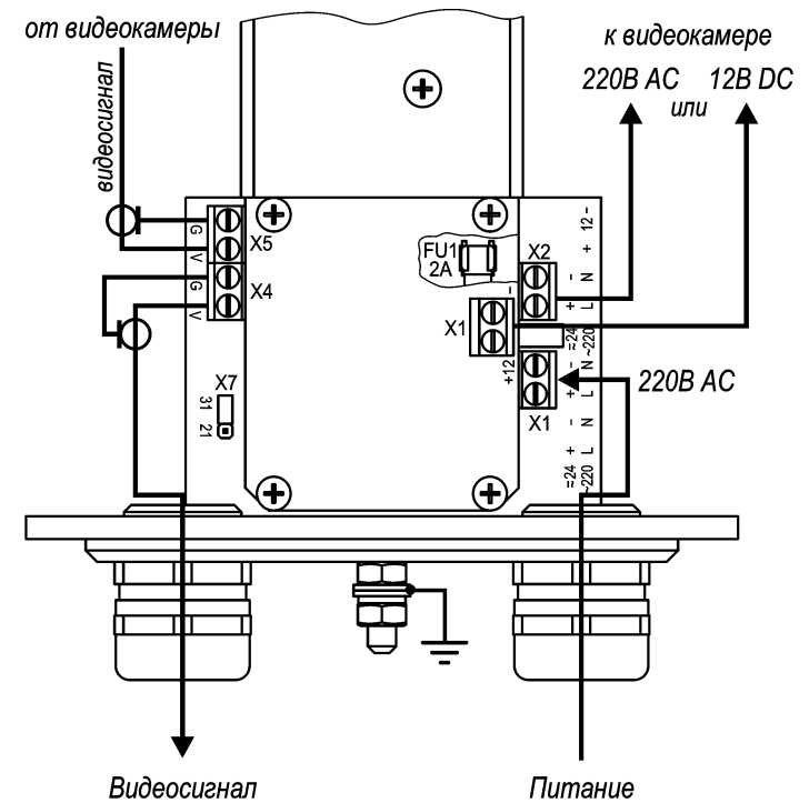
Рис.3 Подключение ТГБ-9У- ~220/12(~220)
