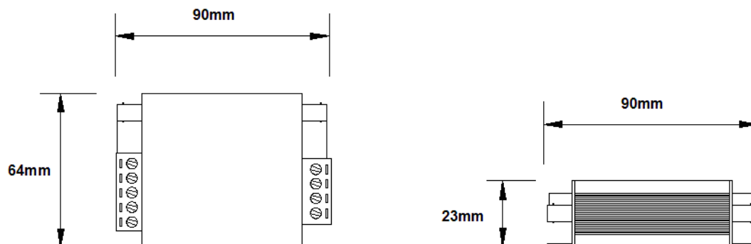
Рис. 2 Габаритные размеры SP-CPD/12-24
