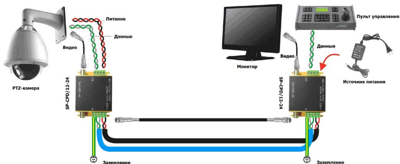
Рис. 3 Подключение SP-CPD/12-24
