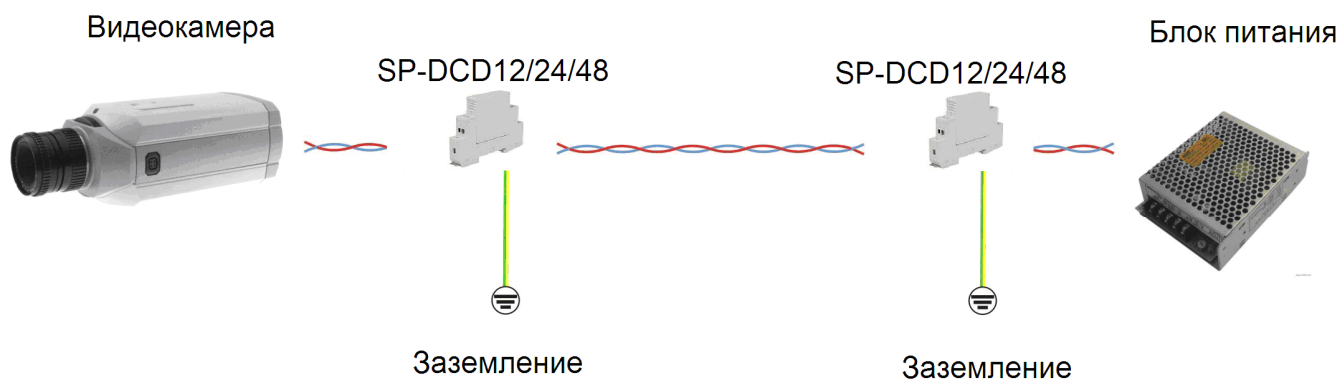
Рис.2 Подключение SP-DCD/12, SP-DCD/24, SP-DCD/48
