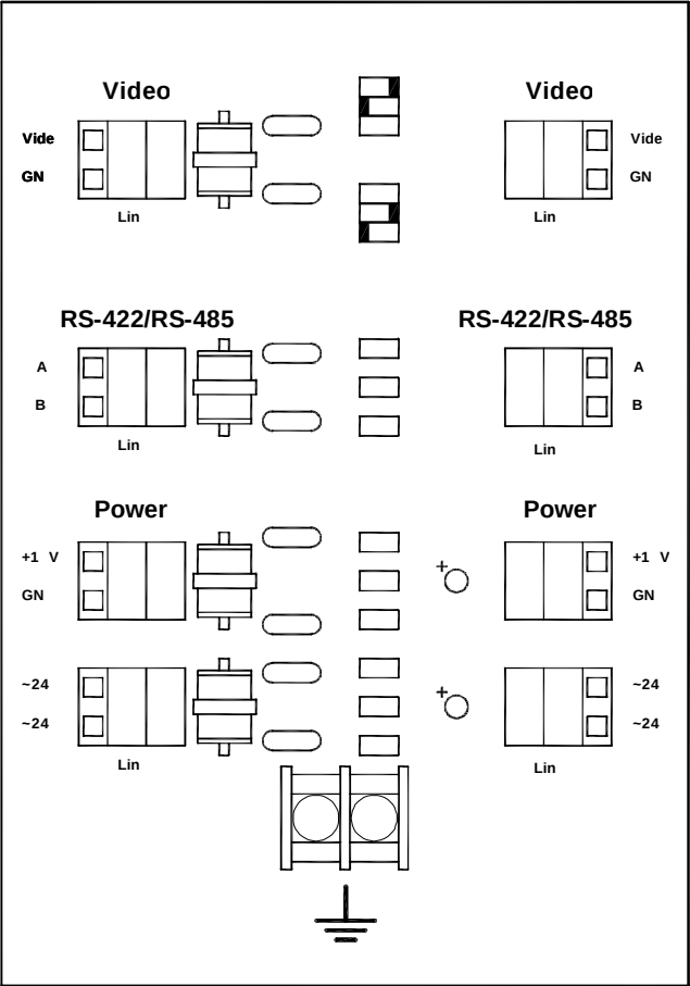
Рис. 1. Схема подключения SVP-24
