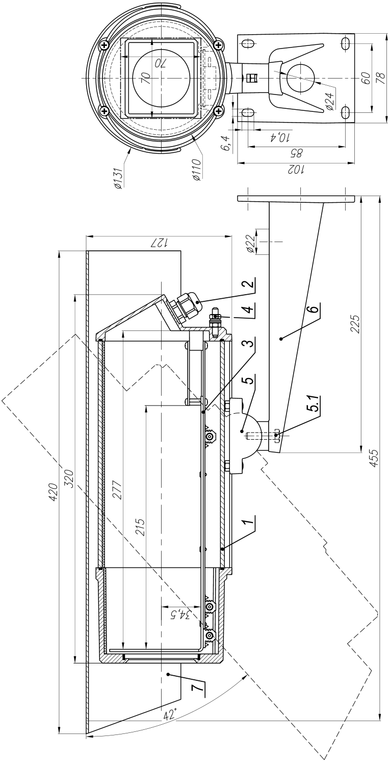
Рис.1 Состав и габаритно-установочные размеры ТГБ-7
