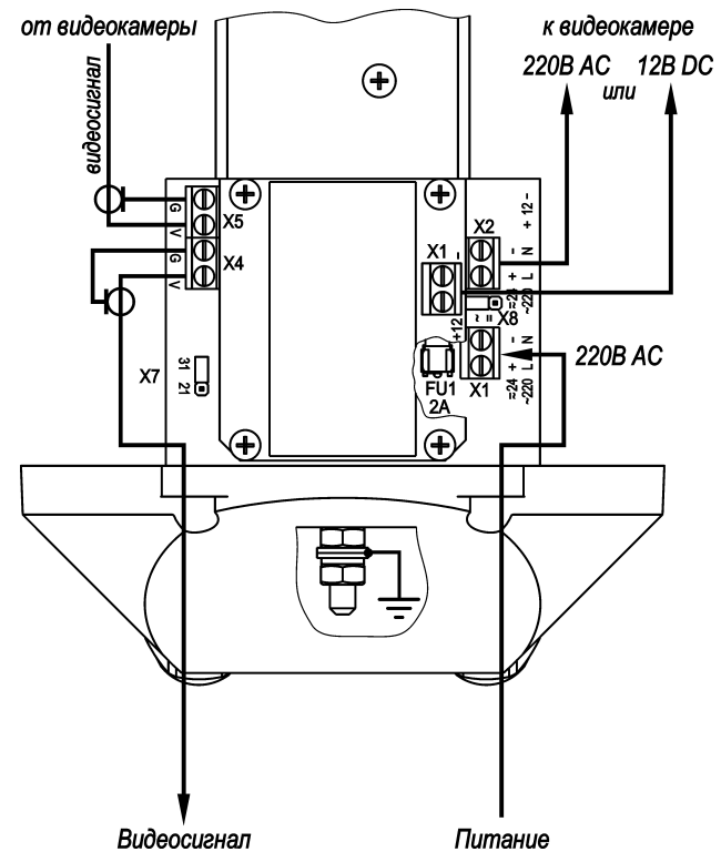
Рис.3 Подключение ТГБ-7- ~220/12(~220)
