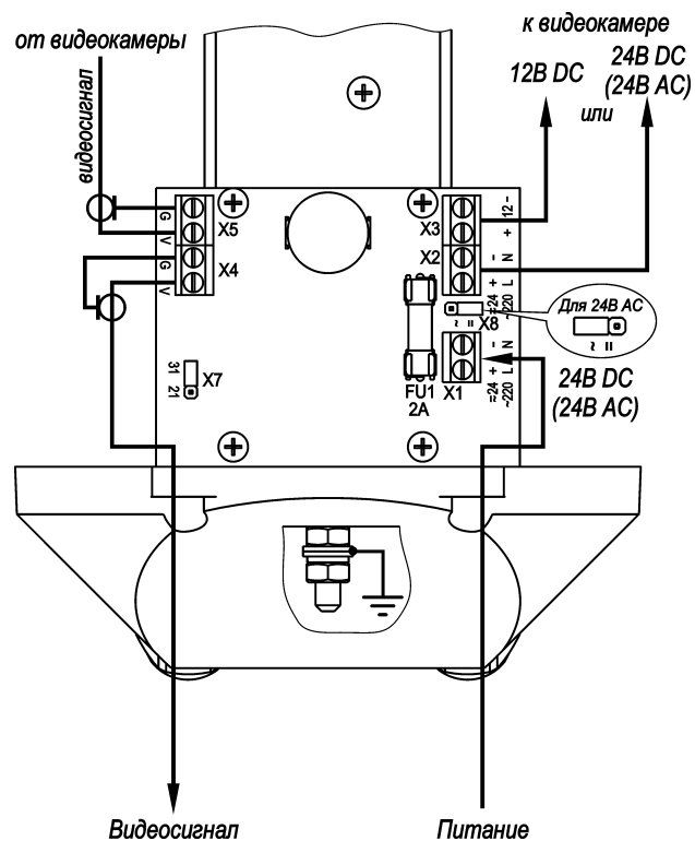
Рис.2 Подключение ТГБ-7-24/12(24); ~24/12(~24)
