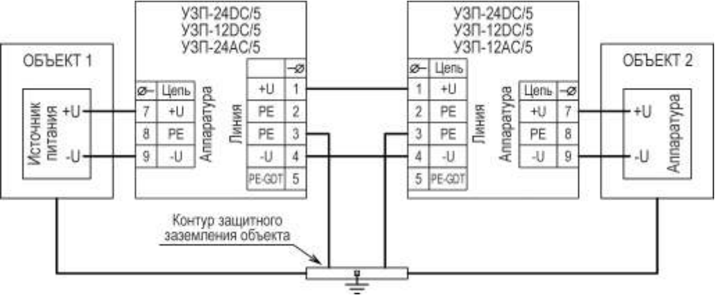
Рис.3 Защита изолированных источников питания устройств, расположенных на одном объекте и имеющих общий контур заземления с системой выравнивания потенциалов
